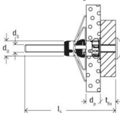
Strichzeichnung
