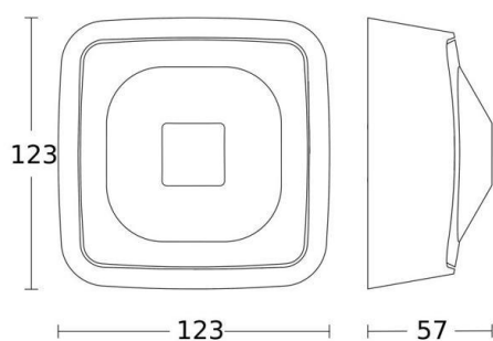
Maßzeichnung
