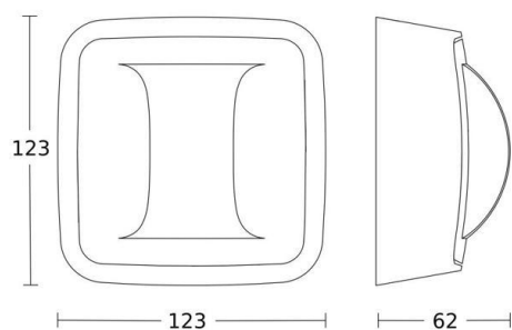
Maßzeichnung
