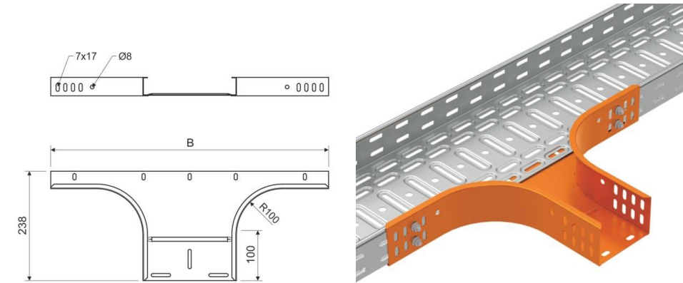
Maßzeichnung
