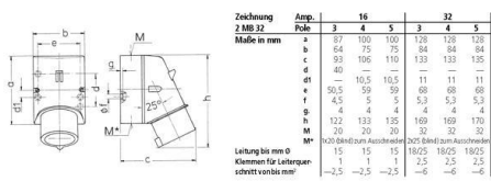
Maßzeichnung
