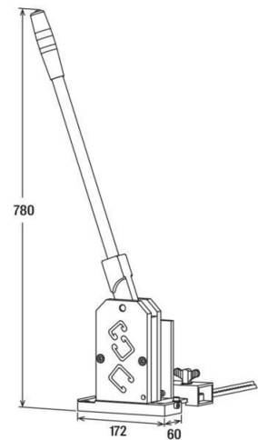
Maßzeichnung
