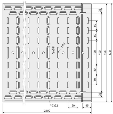
Maßzeichnung
