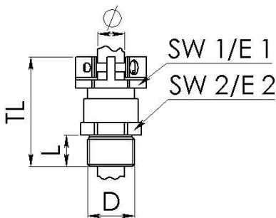
Maßzeichnung
