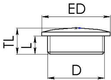
Maßzeichnung
