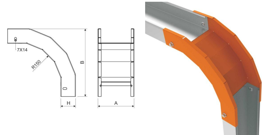
Maßzeichnung
