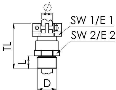
Maßzeichnung
