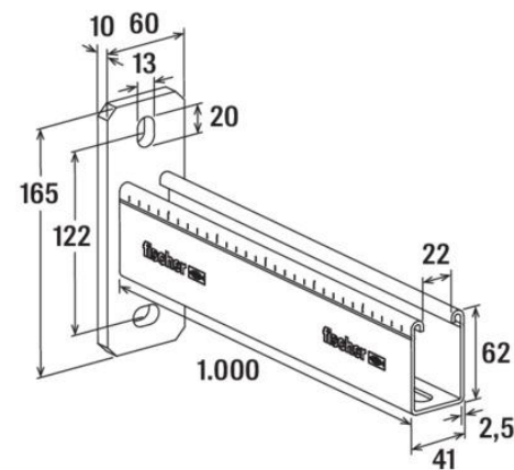
Maßzeichnung
