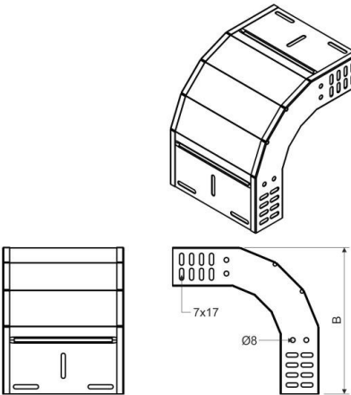
Maßzeichnung
