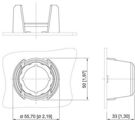
Maßzeichnung
