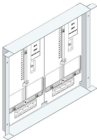
Zählerwanne mit Zählerplatte
