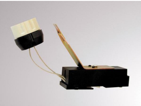
Fassung GU10 mit Klemme & Zugentlastung
