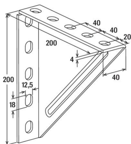
Maßzeichnung
