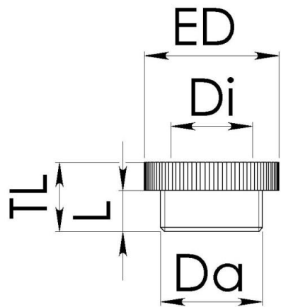
Maßzeichnung
