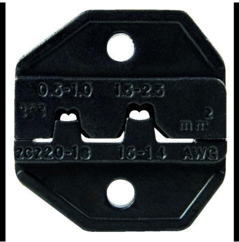
Flachstecker 0,5-2,5
