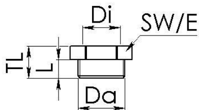
Maßzeichnung
