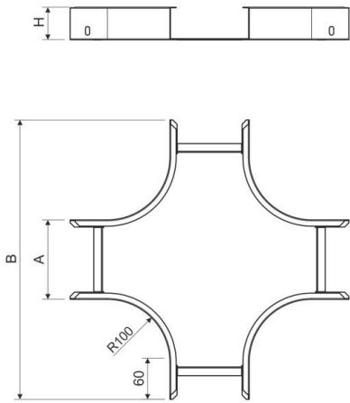
Maßzeichnung
