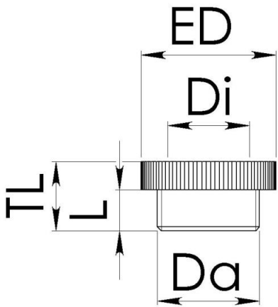
Maßzeichnung
