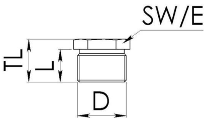
Maßzeichnung
