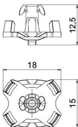
Maßzeichnung
