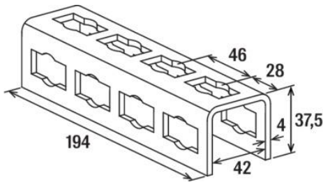
Maßzeichnung
