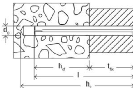
Strichzeichnung
