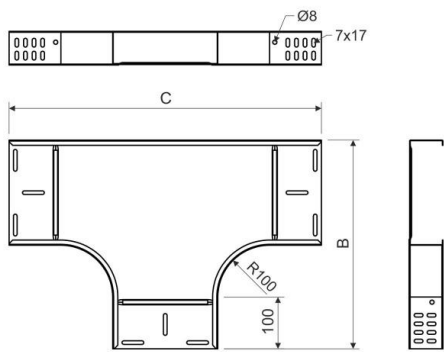
Maßzeichnung
