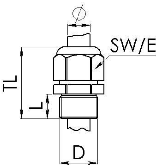
Maßzeichnung
