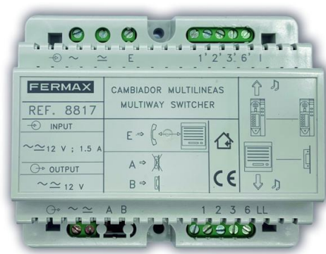
FERMAX Umschaltautomat analog für internen Sprechverkehr
