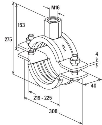
Maßzeichnung
