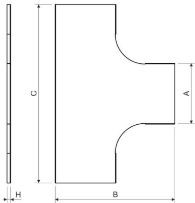
Maßzeichnung
