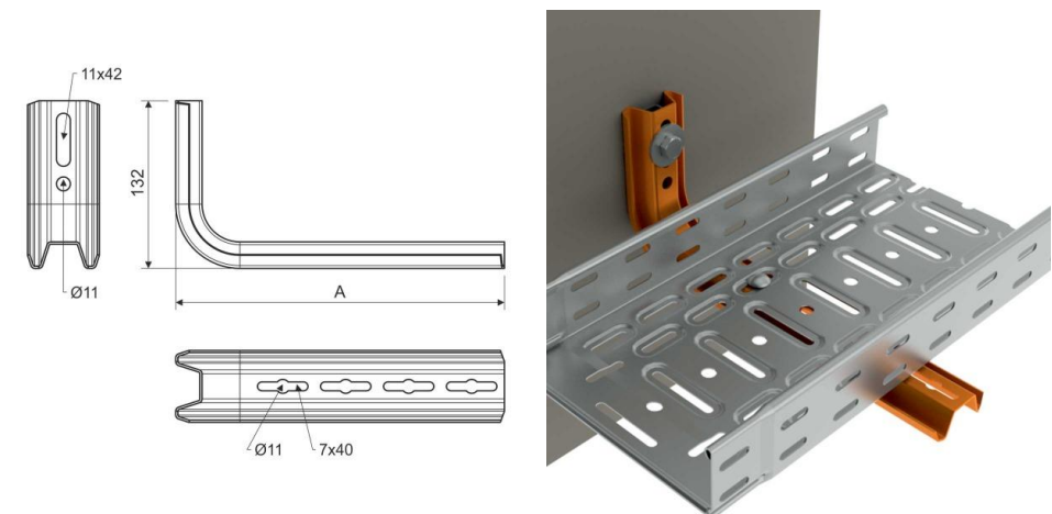
Maßzeichnung
