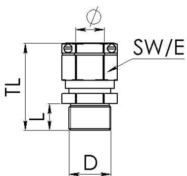
Maßzeichnung
