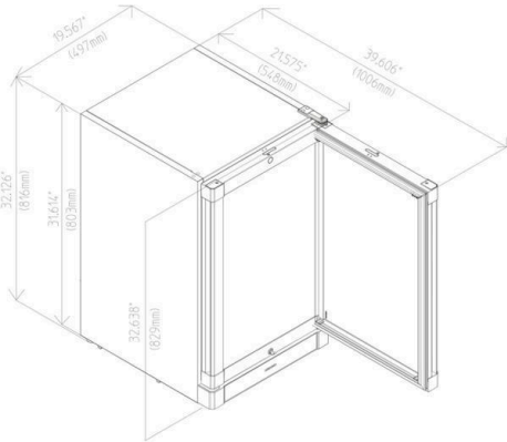
Maßzeichnung
