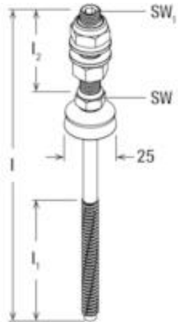
Strichzeichnung
