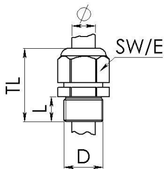
Maßzeichnung
