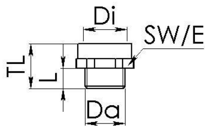
Maßzeichnung
