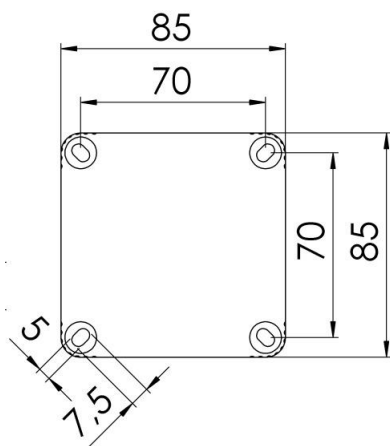
Maßzeichnung
