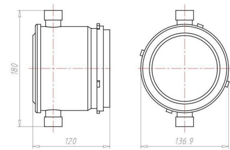
Maßzeichnung
