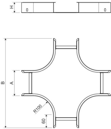
Maßzeichnung
