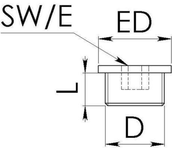
Maßzeichnung
