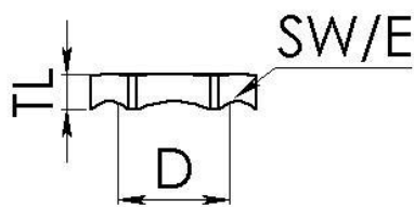
Maßzeichnung
