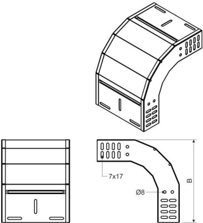
Maßzeichnung
