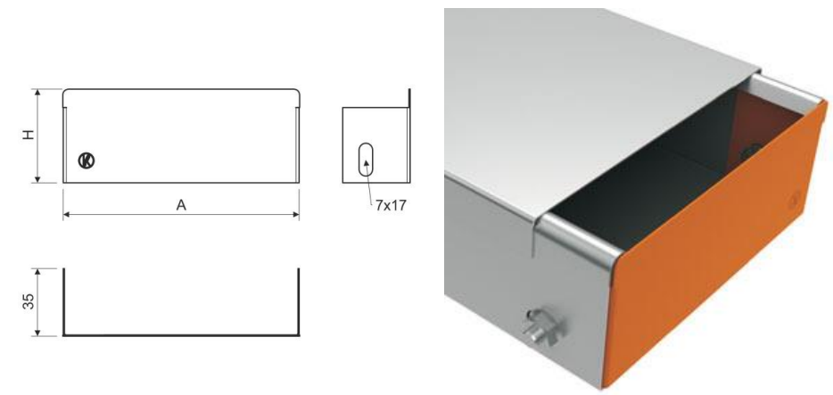
Maßzeichnung
