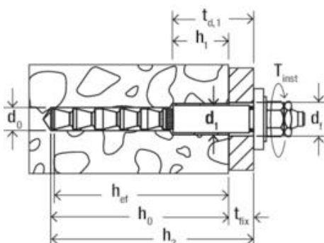
Strichzeichnung
