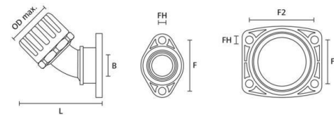
Maßzeichnung
