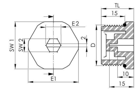
Maßzeichnung
