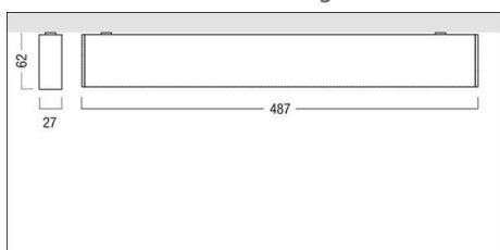
Maßzeichnung
