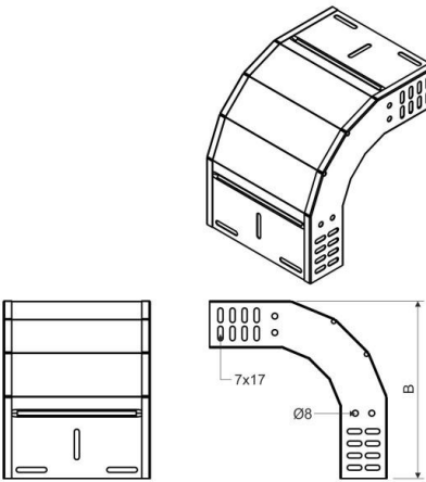
Maßzeichnung
