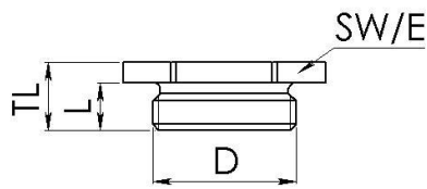
Maßzeichnung
